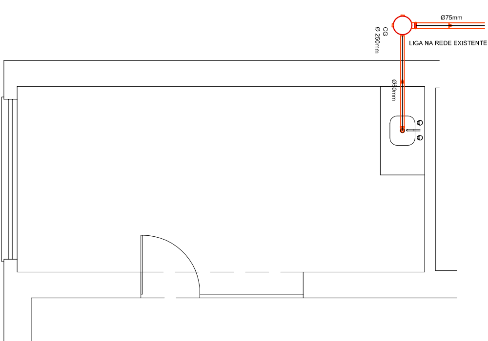
ESGOTO SANITÁRIO - BLOCO B-1 Esc. 1/50
