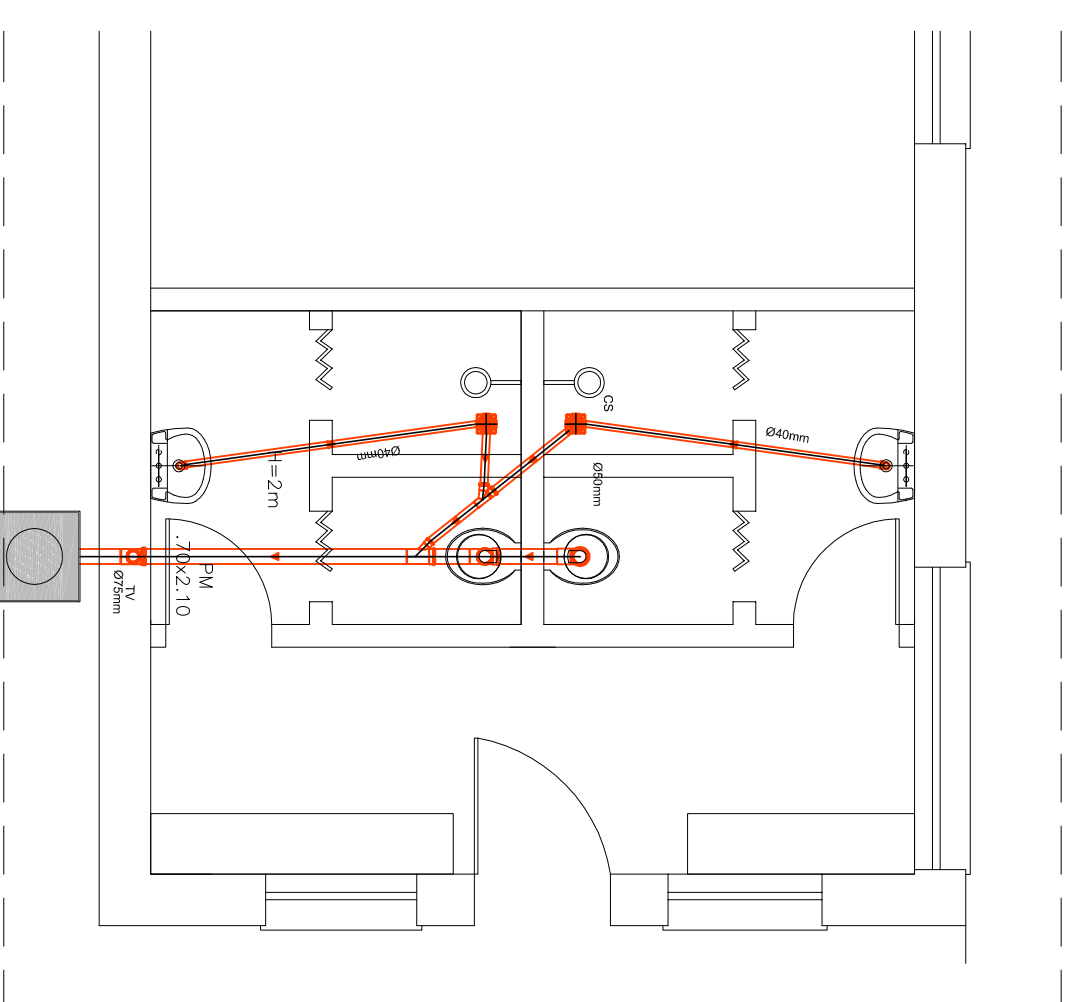
ESGOTO SANITÁRIO - BLOCO B-2 Esc. 1/50
