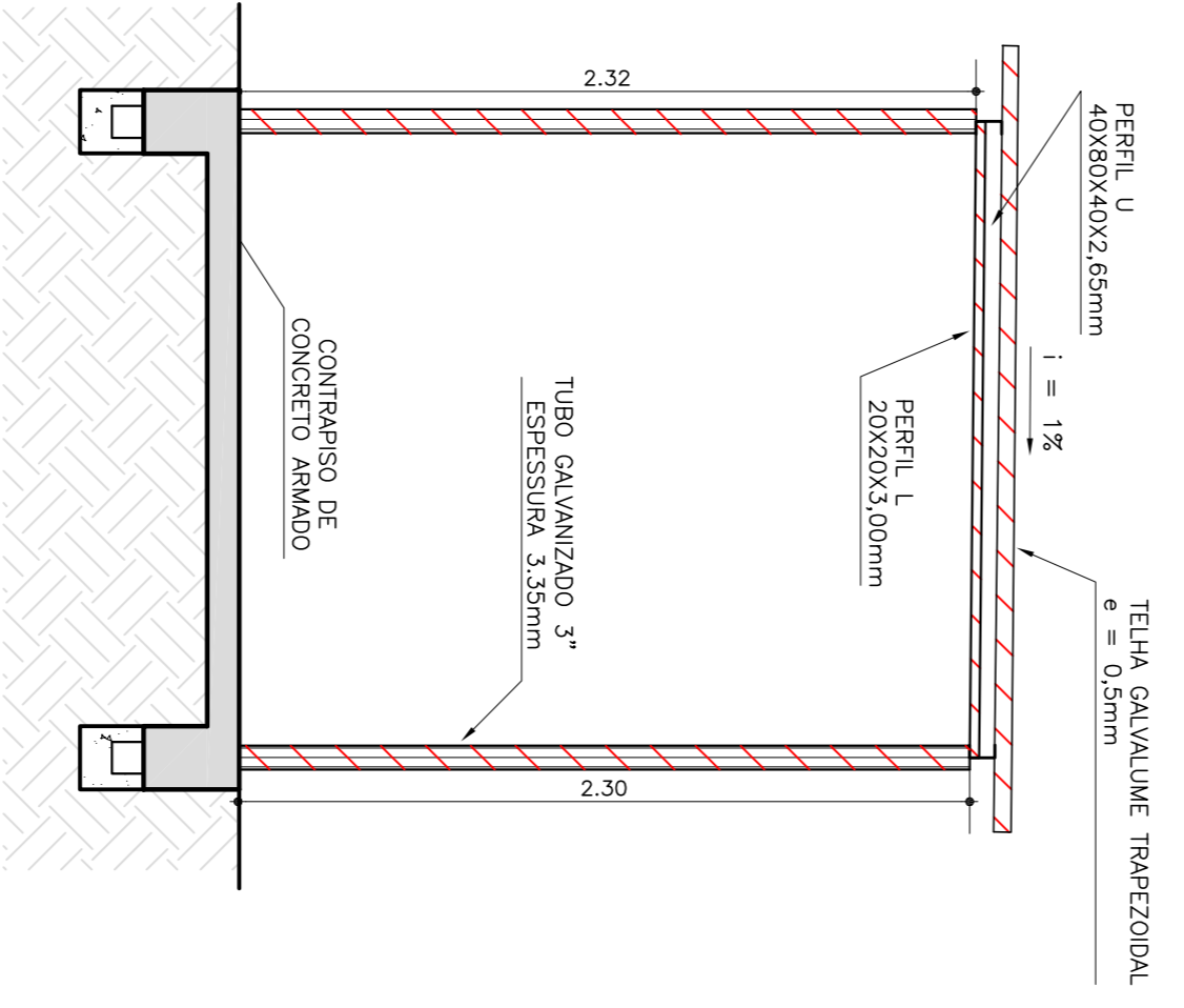
CORTE A-B ESCALA 1/25
